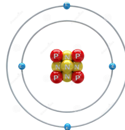
ATOMO DI BERILLIO
