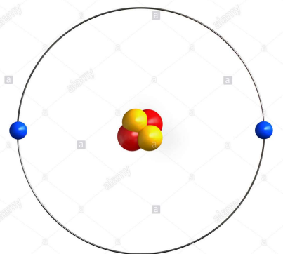
ATOMO DI ELIO
