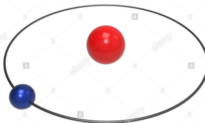
ATOMO DI IDROGENO
